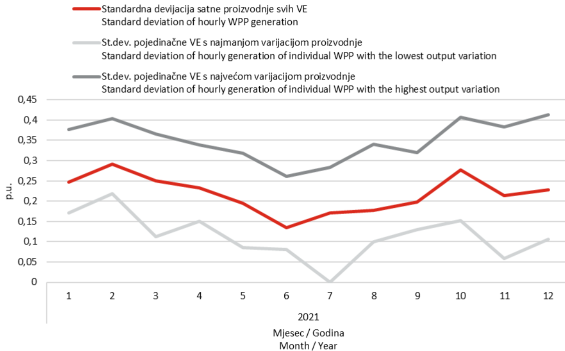
Slika 5 Standardna devijacija satne proizvodnje vjetroelektrana u jediničnim vrijednostima
