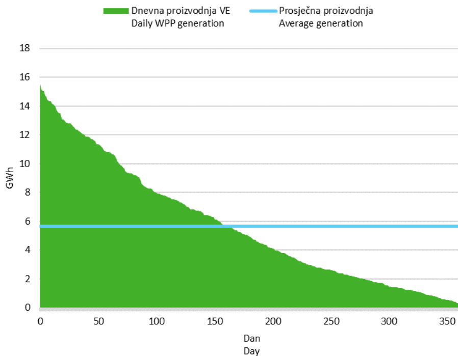
Slika 7 Krivulja trajanja dnevne proizvodnje vjetroelektrana Figure 7 Average daily WPP generation duration curve
