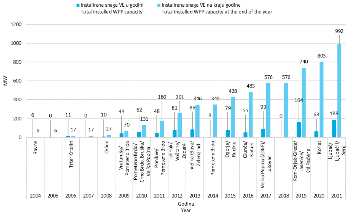
Slika 2 Vremenska dinamika izgradnje VE u Hrvatskoj Figure 2 Time horizon of wind power plant construction in Croatia
